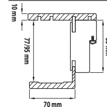
TELAIO TECNO DA 80 mm TECNO FRAME 80 mm
