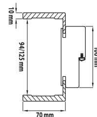
TELAIO PLANAR DA 113 mm PLANAR FRAME 113 mm
