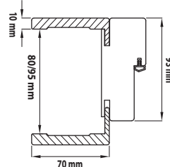
TELAIO PLANAR DA 93 mm PLANAR FRAME 93 mm
