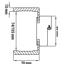
TELAIO PLANAR DA 93 mm PLANAR FRAME 93 mm
