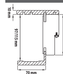
TELAIO TECNO DA 100 mm TECNO FRAME 100 mm
