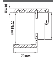
TELAIO TECNO DA 80 mm TECNO FRAME 80 mm
