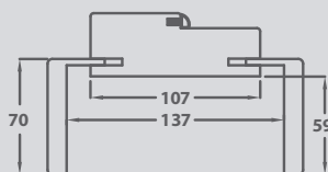
telaio FLAT di serie standard FLAT frame
