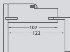
telaio ZEN ZEN frame
