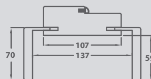
telaio FLAT FLAT frame
