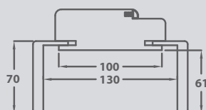
telaio standard standard frame
