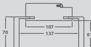
telaio di serie standard frame
