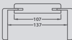
telaio standard per passata standard frame without door
