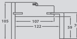
telaio ZEN ZEN frame
